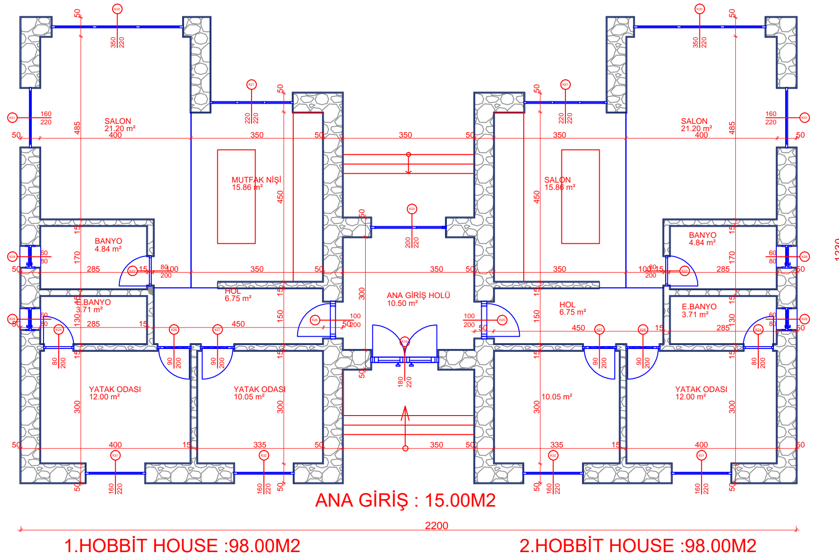
ZEMİN KAT PLANI
